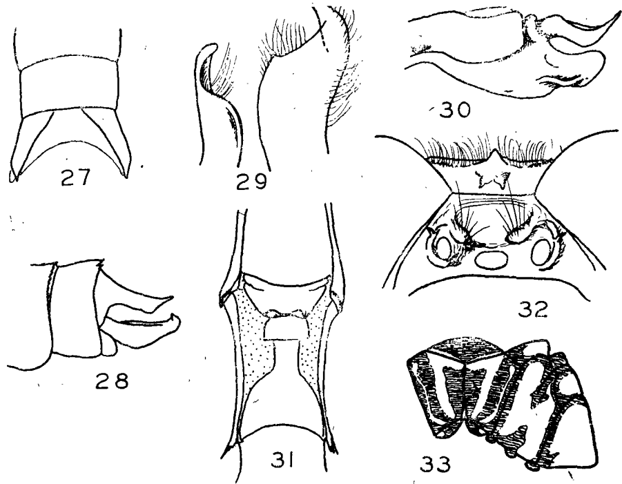
圖 27—33 Gomphus perluetus , sp. nov.—— 27. 肛附器, 背面觀。 28. 肛附器, 側面觀。 29. 前後鈎片, 側面觀。 30. 陽莖末端, 側面觀。 31. ♀, 下生殖板及第 9 節腹板。 32. ♀, 頭部, 側面觀。 33. 合胸色彩。
