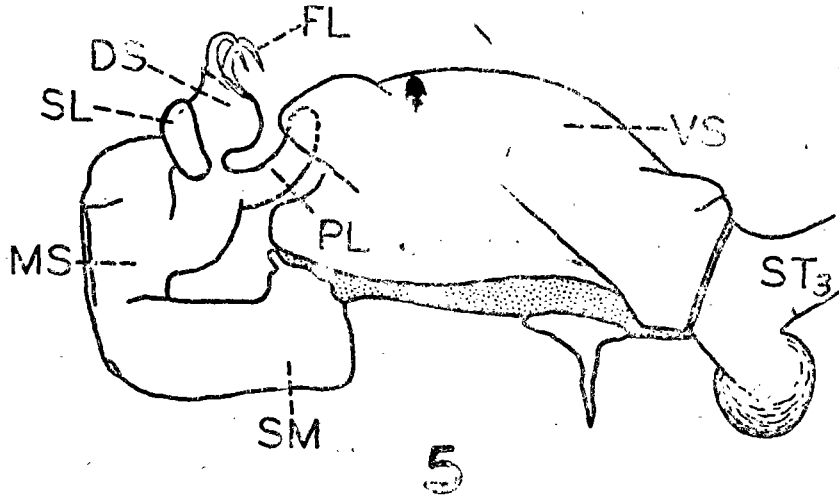
圖 5 Onychogomphus ardens Needham, ♂, 陽莖, 側面觀。 DS—末節。 FL—鞭。 MS—中節。 PL—後葉。 SL—鱗狀瓣。 SM—鱗瓣。 VS—陰囊。 ST 3 —腹部第 3 節腹板。
