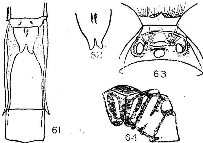
圖 61—64 Gomphus szekuanicus , sp. nov., ♀—— 61. 下生殖板及腹末 3 節，腹面觀。 62. 下生殖板，根據福建的副模標本所繪。 63. ♀，頭部，背面觀。 64. 合胸色彩。
