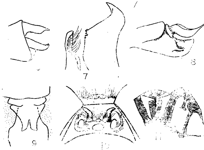
圖6—11 Gomphus cuneatus Needham——6. 肛附器, 側面觀。7. 前後鉤片, 側面觀。 8. 陽莖末端, 側面觀。9. ♀, 下生殖板。10. ♀, 頭部, 背面觀。11. 合胸色彩。
