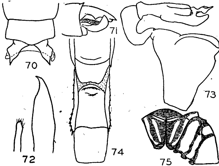
圖 70—75 Gomphus clathratus Needham —— 70. 肛附器，背面觀。71. 肛附器，側面觀。72. 前後鈎片，側面觀。73. 陽莖，側面觀。74. 下生殖板及腹末2節，腹面觀。75. 合胸色彩。
