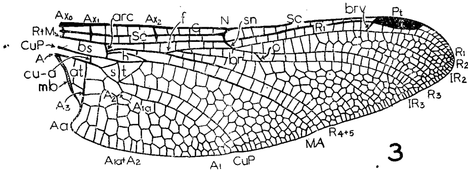
圖 2—3. Gomphus cuneatus Needham, ♂, 翅, (除若干翅脈及翅室加以註解外, 各主要縱脈, 不另說明) 2. 前翅。 3. 後翅。 Aa—臀角。 Ax 0 , Ax 1 , Ax 2 —翅基, 第一及第二原始節前橫脈。 arc—弓脈。 at—臀三角室。 br—橋脈。 brv—支持脈。 bs—基室。 cu-a—肘臀脈。 f—叉脈。 h—上三角室。 mb—小膜瓣。 N—翅結。 o—斜脈。 Pt—翅痣。 s—下三角室。 sn—亞翅結。 t—三角室。
