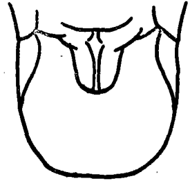
圖 83 Gomphus somnolens Needham 下生殖板(做 Needham 原圖)
