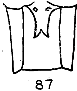
圖 87 Gomphus torpens Needham, 下生殖板。(做 Needham 原圖)
