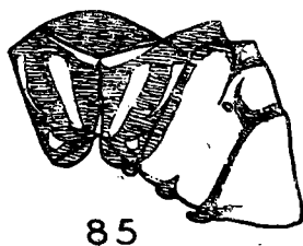
圖 85-86 Gomphus endicotti Needham — 85. 合胸色彩, 根據完模標本所繪。 86. 下生殖板做 Needham 原圖。
