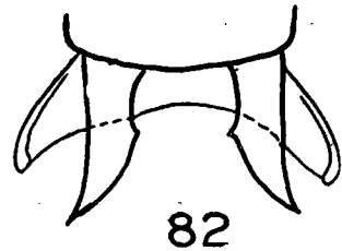
圖 82 Gomphus corniger Morton 肛附器, 背面觀。(仿 Morton 原圖)
