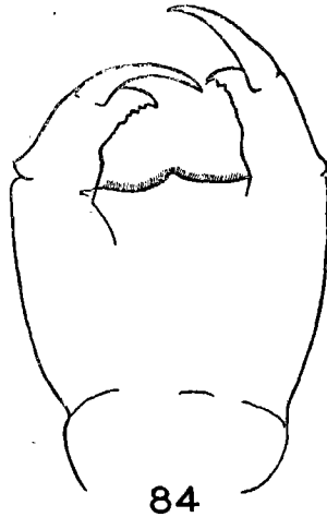
圖 84 Gomphus somnolens Needham 稚蟲下唇 (做 Needham 原圖)
