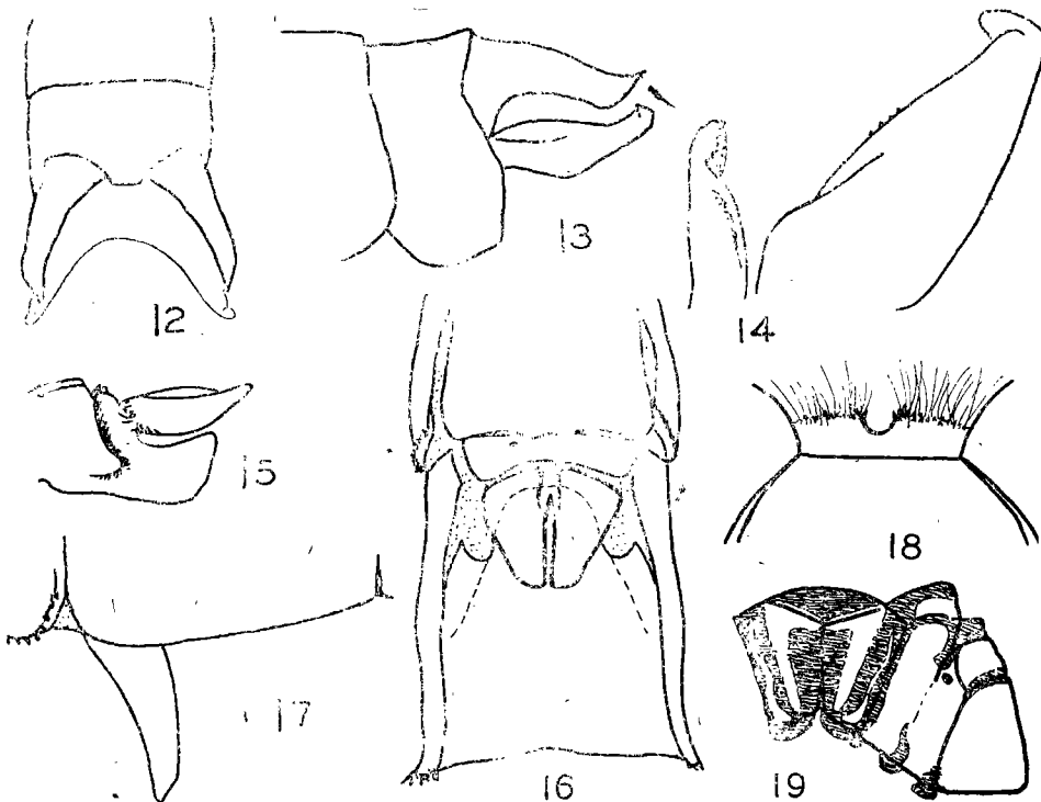
圖 12—19 Gomphus septimus Needham——12. 肛附器，背面觀。 13. 肛附器，側面觀。14. 前後鈎片，側面觀。15. 陽莖末端，側面觀。16. ♀ 下 生殖板及第 9 節腹板。17. ♀ 下生殖板，側面觀。18. ♀ 後頭緣，前面觀。 19. 合胸色彩。
