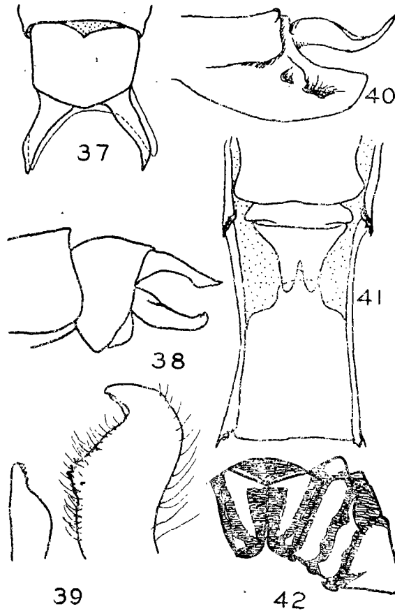
圖 57-42. Gonplius pacificus , sp. nov. — 57. 肛附器，背面觀。 58. 肛附器，側面觀。 59. 前後鈎片，側面觀。 40. 陽莖末端，側面觀。 41. ♀，下生殖板及第 9 節腹板。 42. 合胸色彩。
